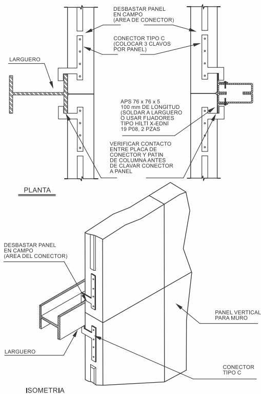
Detalle 5: Fijación de paneles verticales para muro a estructura de acero con conector Tipo "C".
