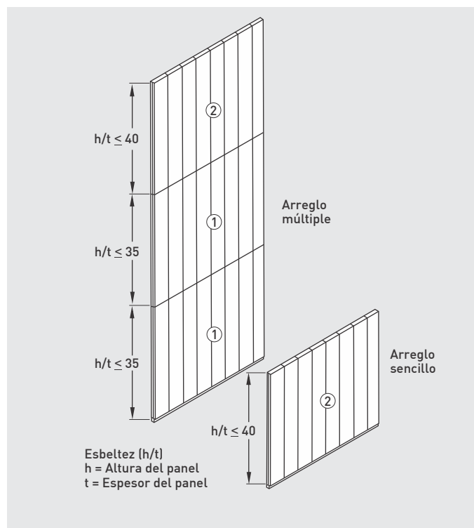
Fig. 4: Arreglo vertical de paneles Hebel para muro.
