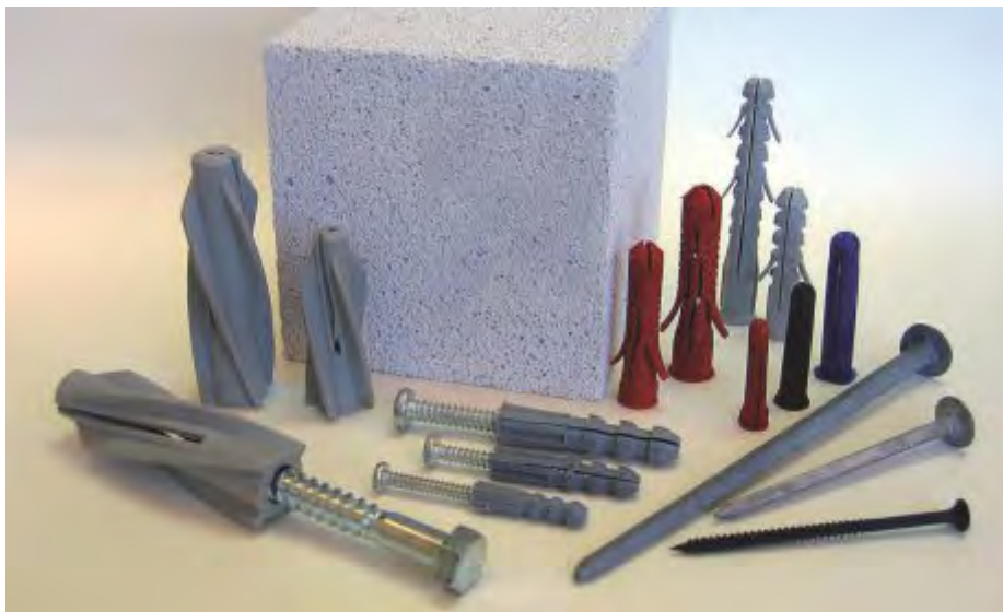
Fig. 32: Taquetes recomendados para Concreto Celular Hebel.
