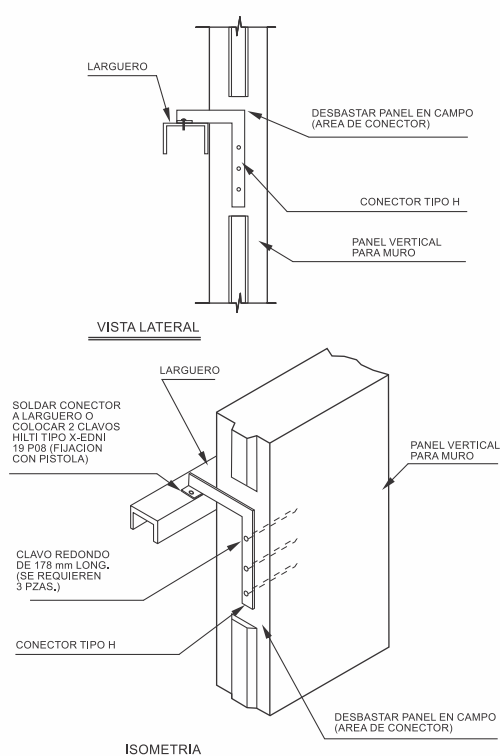
Detalle 6: Fijación de paneles verticales para muro a estructura de acero con conector Tipo "H".
