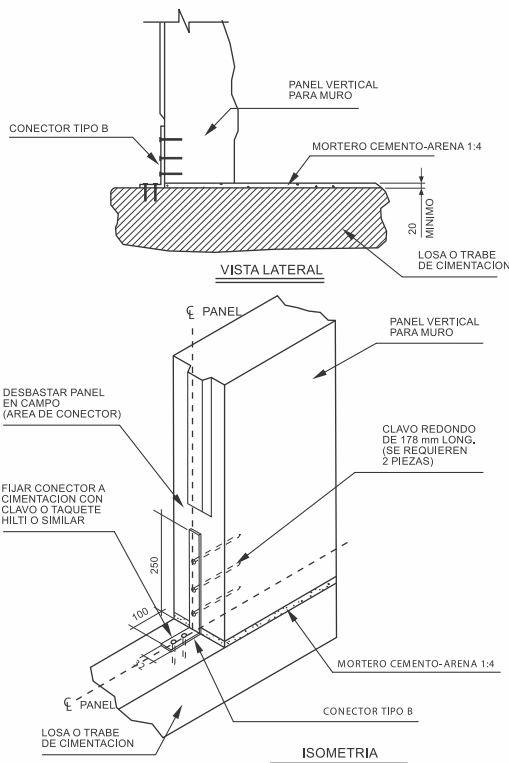
Detalle 7: Fijación de paneles verticales a trabe de concreto con conector Tipo "B".
