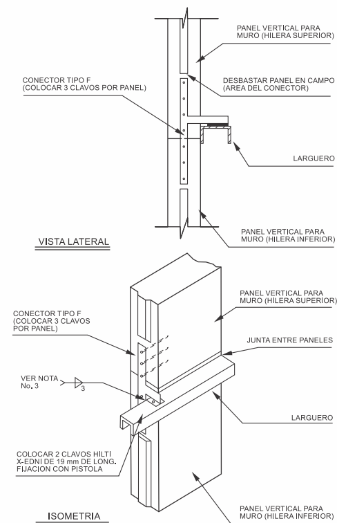
Detalle 8: Fijación de paneles verticales para muro a estructura de acero con conector Tipo "F".
