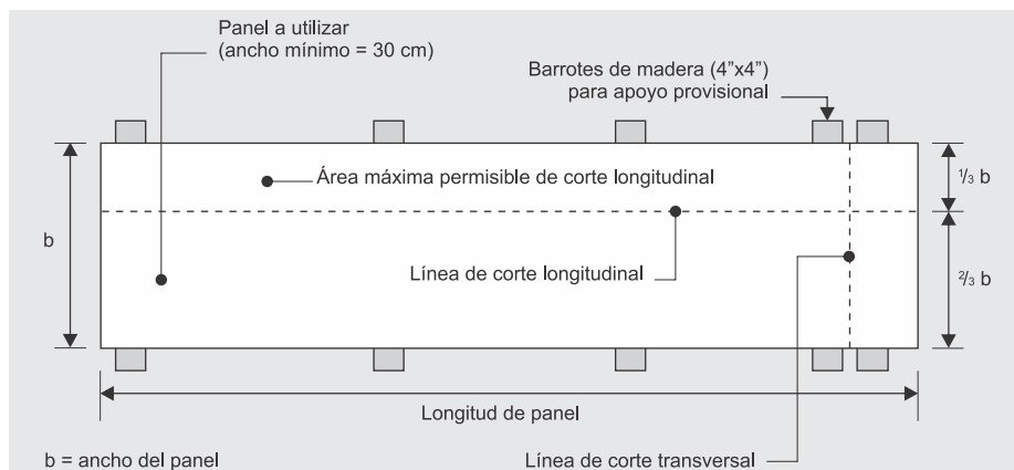
Fig. 28: Área permisible de corte.
